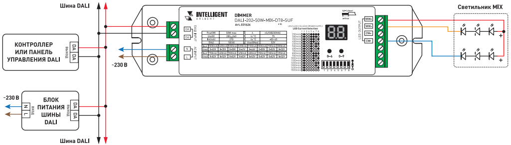
Рисунок 2. Пример схемы подключения диммера DALI-202-50W-MIX-DT8-SUF по трехпроводной схеме
