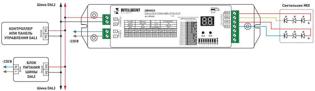
Рисунок 1. Пример схемы подключения диммера DALI-202-50W-MIX-DT8-SUF по четырехпроводной схеме
