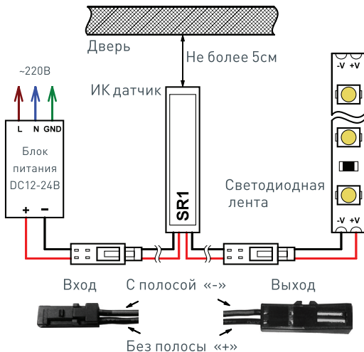
Рис.1. Схема подключения.
